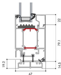
Version 67PL seuil étanche
