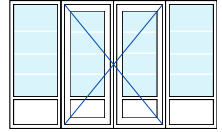
Ensemble composé porte balcon 2 ouvrants + fixes latéraux avec soubassement
