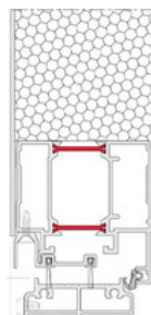
Version 67PL monobloc
