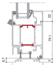
Version 67PL seuil plat
